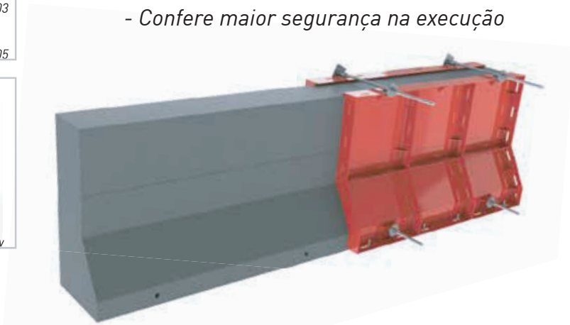
01 - New Jersey Angular e New Jersey Reta 02 - Clips 03 - Perfil VL5 04 - Barra de Ancoragem 05 - Porca de Ancoragem 06 - Othal
